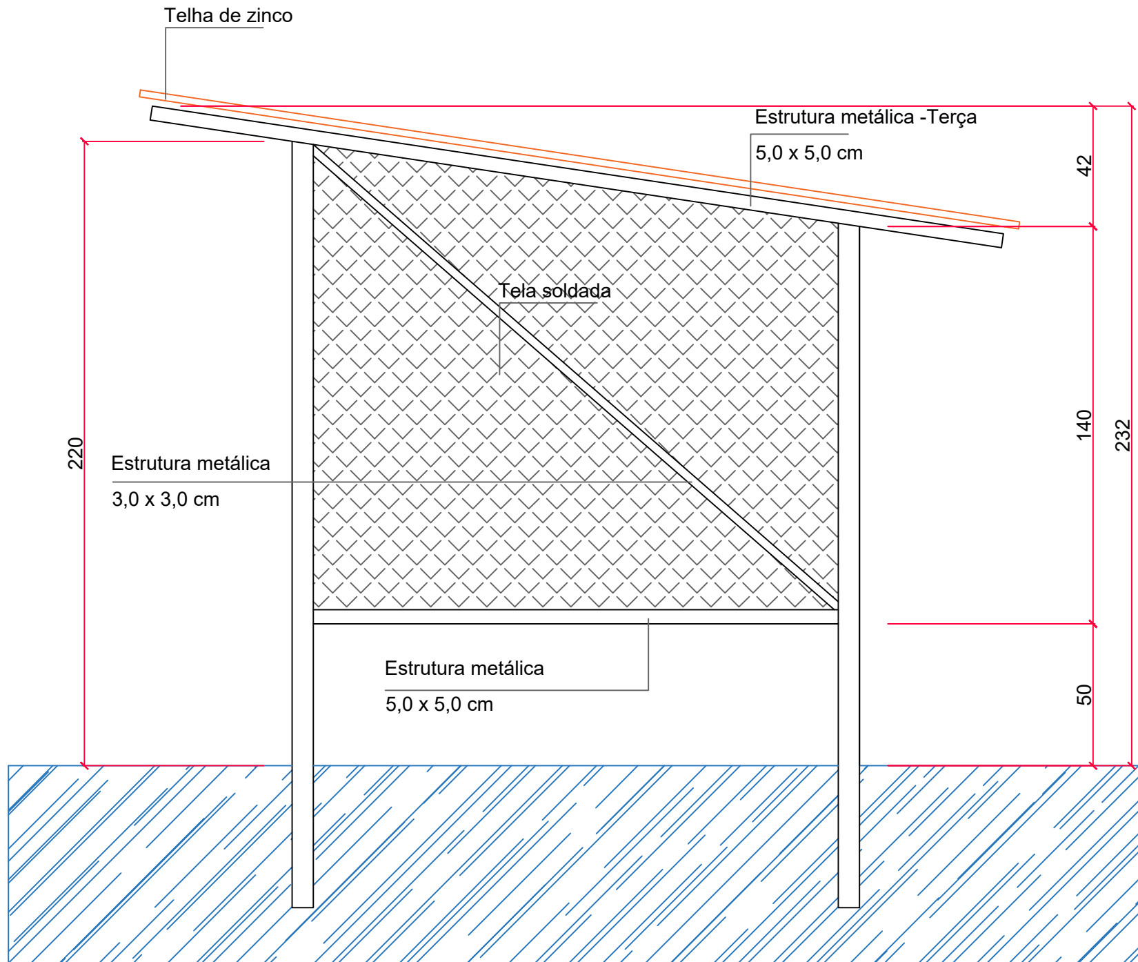
Corte Longitudinal AA
