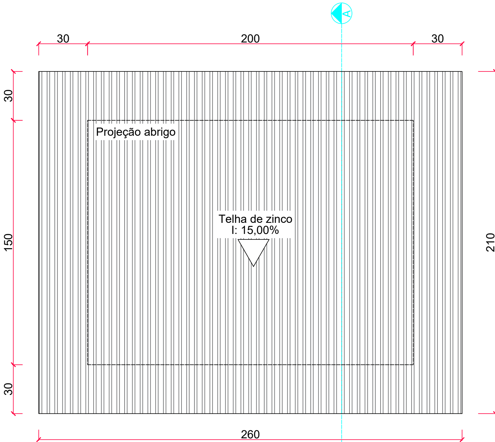
Planta de Cobertura
