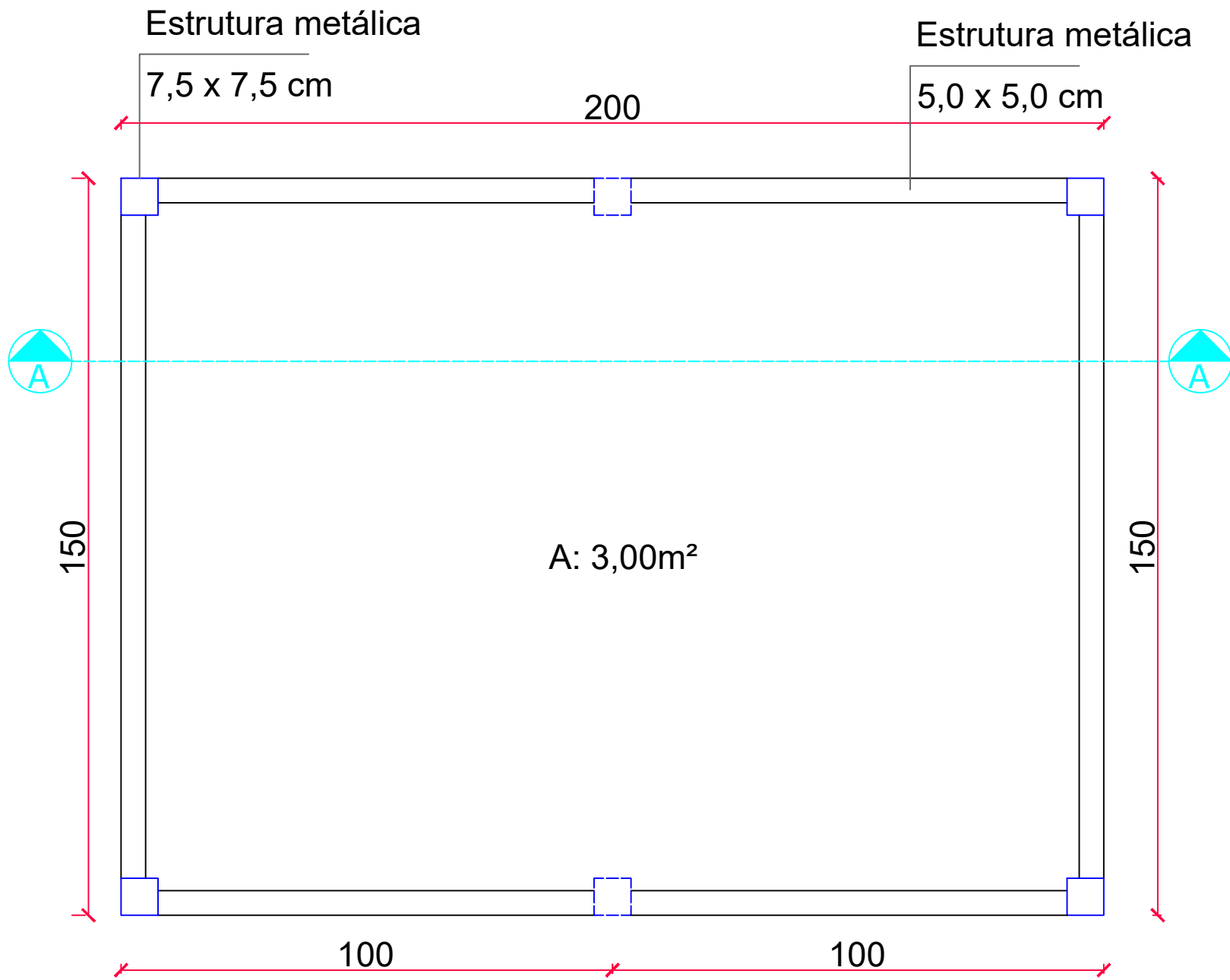
Planta Baixa
